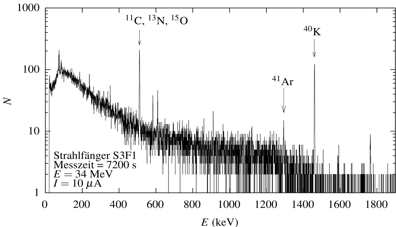
Abbildung 6: Gamma-Spektrum zur Identifizierung und Aktivitätsbestimmung der Radionuklide ^{11}\text{C} , ^{13}\text{N} , ^{15}\text{O} bei 511 keV (Annihilationsstrahlung) und ^{41}\text{Ar} bei 1294 keV in einer Luftprobe der Beschleunigeranlage S-DALINAC (TU Darmstadt).
