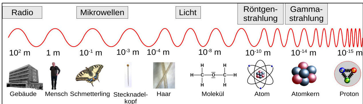
Abbildung 2: Wellenlängen im elektromagnetischen Spektrum im Vergleich mit makroskopischen und mikroskopischen Objekten unserer Welt.
