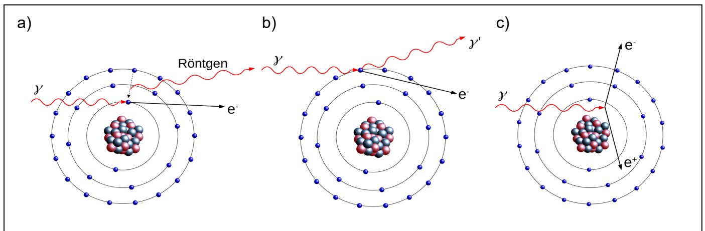
Abbildung 4: Prinzipskizzen zum Photoeffekt a), Compton-Effekt b) und zur Paarbildung c).
