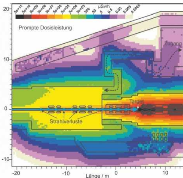
19 Abschirmrechnungen für den Target- und Vortarget-Bereich des SuperFRS (Supraleitender Fragment Separator)
